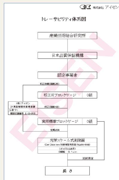
トレーサビリティ体系図 Traceability system diagram
